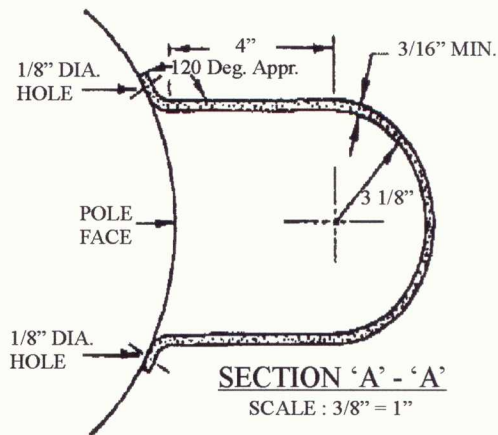
CONDUIT
